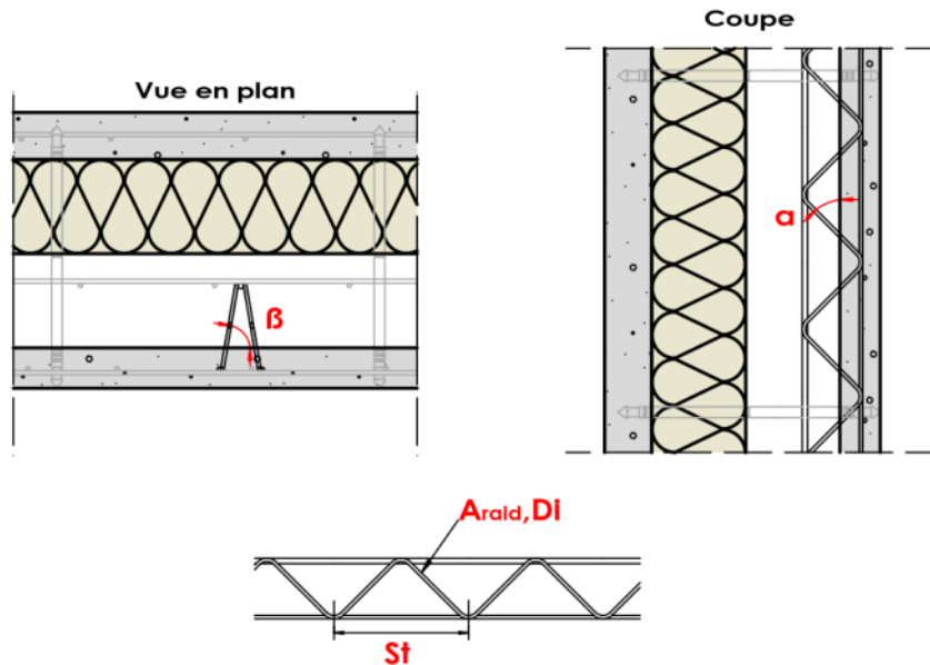
Figure 89 : Géométrie des raidisseurs type treillis Warren
