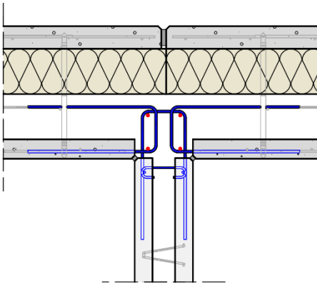
Figure 38 : Liaison verticale en T encastrée – Type Ev5
