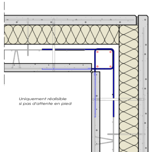
Figure 47 : Liaison d'angle couturée en zone sismique avec chaînage
