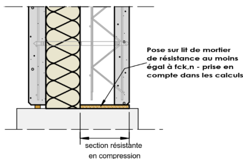
Figure 12 : Section résistante en compression en fonction du type d'appui
