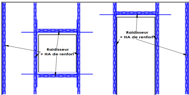
Figure 14 : Réalisation de chaînage en (i)Premur A2C
