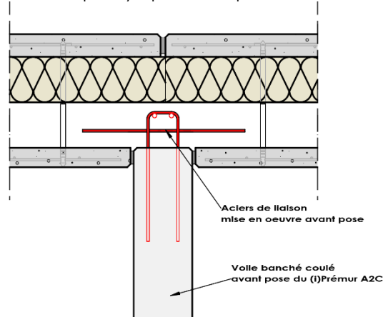
Figure 32 : Liaison en T entre un (i)Premur A2C et un mur coulé en place.
