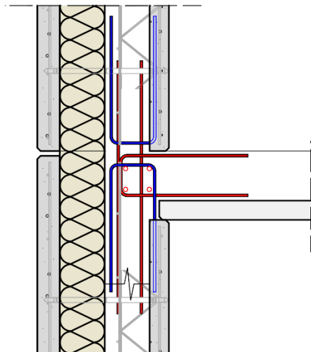
Figure 30 : Liaison dalle/ (i)Premur A2C encastrée
