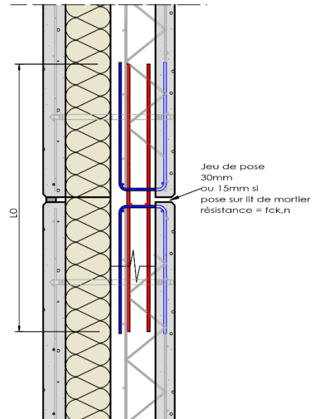
Figure 41 : Liaisons horizontales encastrées – Type Eh1
