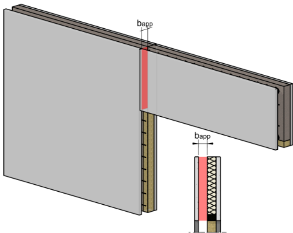
Figure 54 : Appui de poutre → Cas 1
