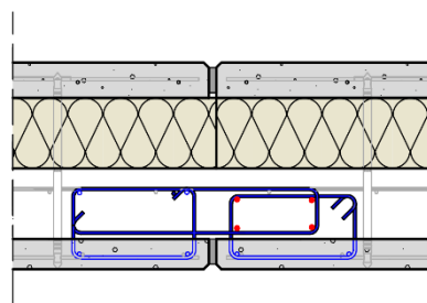
Figure 35 : Joint vertical encastré – Type de type Ev1
