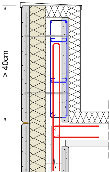
Figure 59 : Acrotère haut constitué d'un (i)Premur A2C rapporté
