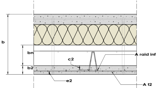
Figure 13 : Enrobages des raidisseurs
