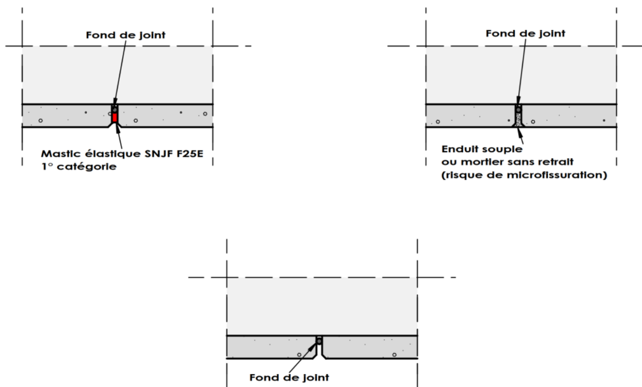
Figure 70 : Traitement du joint INTERIEUR entre (i)Premur A2C
