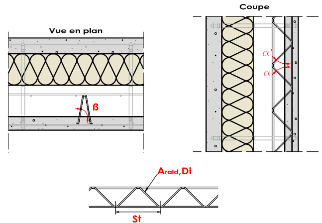
Figure 16 : Définition des raidisseurs de l'(i)Premur A2C
