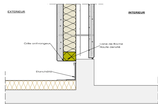
Figure 64 : Liaison (i)Premur A2C/Terrasse
