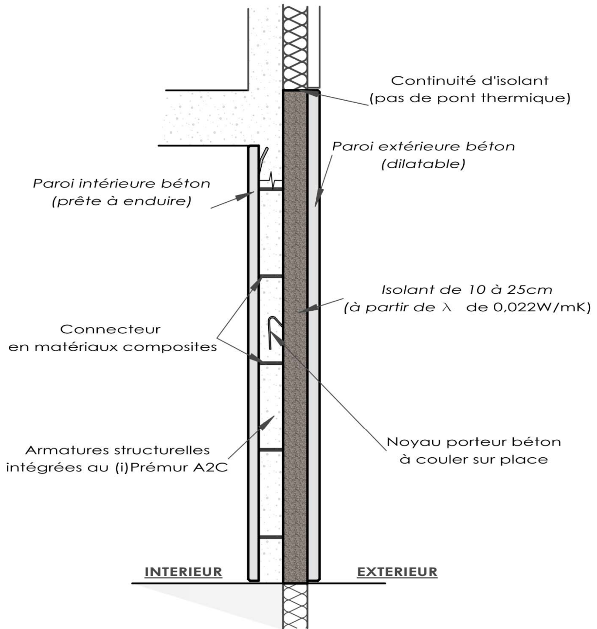
Figure 93 : Coupes verticales courantes de l'(i)Premur A2C
