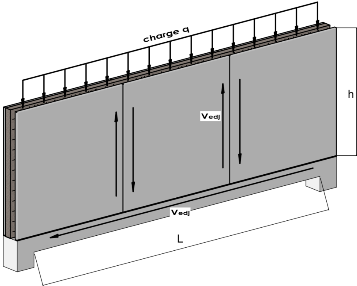
Figure 76 : Effort sollicitant dans le cas d'une poutre-voile
