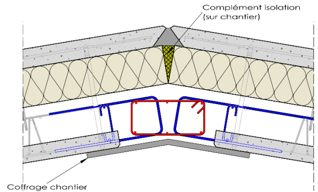
Figure 40 : Liaison verticale d'angle encastrée
