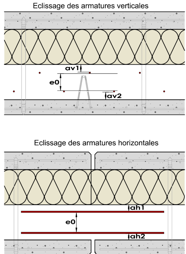
Figure 19 : Eclissage des armatures dans l'(i)Premur A2C
