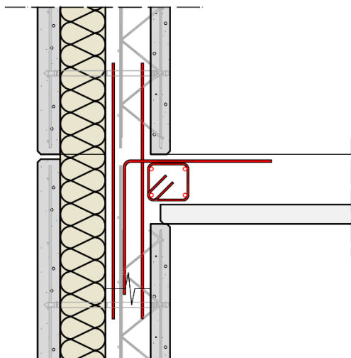
Figure 27 : Liaison rotulée de l'(i)Premur A2C avec une dalle
