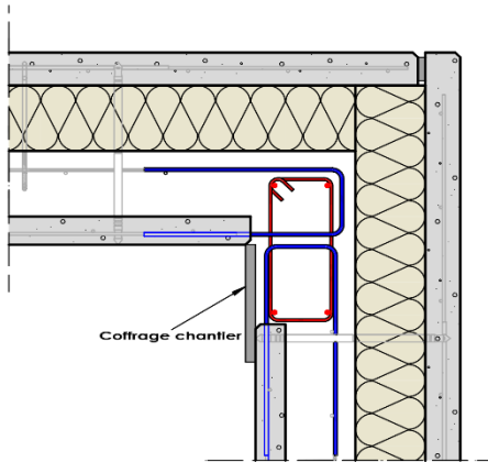
Figure 37 : Liaisons d'angle encastrées – Type Ev3 (en haut) et Ev4 (en bas)
