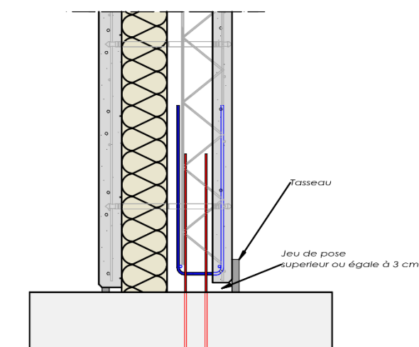
Figure 25 : Encastrement de l'(i)Premur A2C/radier → Liaison de type Er1
