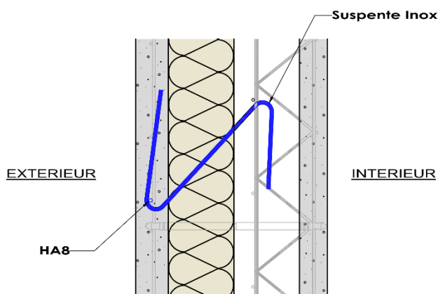
Figure 7 : Coupe sur les suspentes Inox de l'(i)Premur A2C
