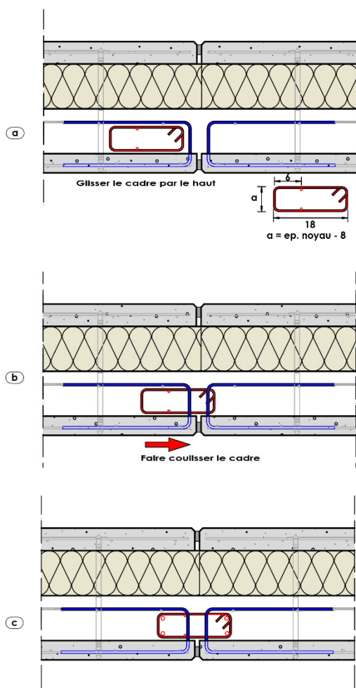
Figure 34 : Liaison verticale couturée droite – Type C1
