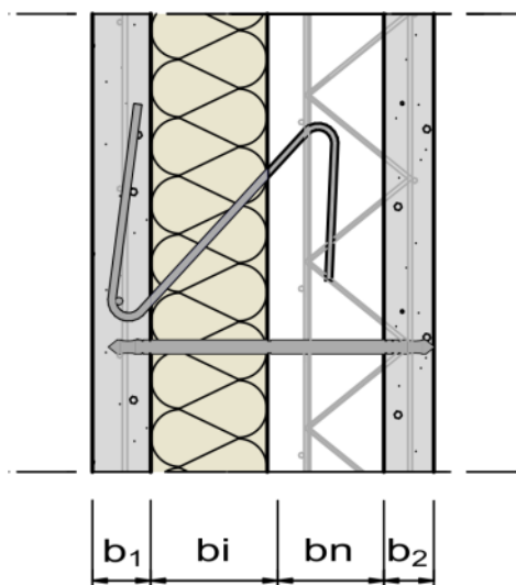
Figure 57 : Repérage des épaisseurs unitaires d'un (i)Premur A2C
