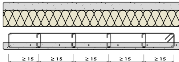
Figure 52 : Section de poteau fortement chargé
