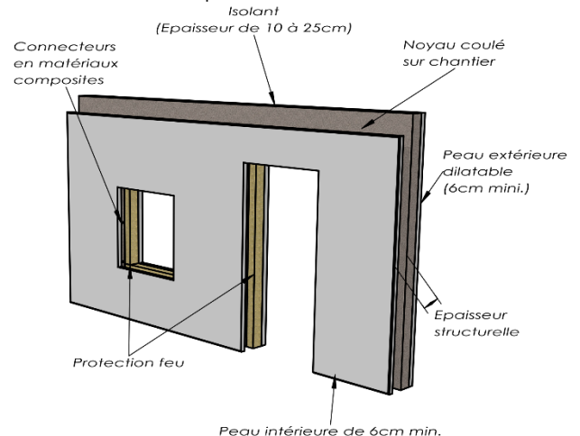
Figure 1: Définition de l'(i)Premur A2C
