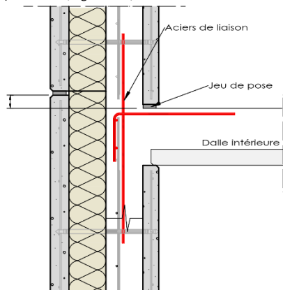
Figure 65 : Détails sur joints horizontaux : paroi extérieure plus haute de 15 mm vis-à-vis du plancher
