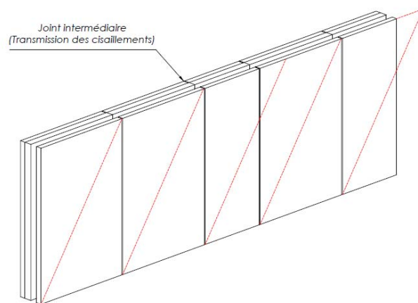
Figure 43 : Comportement monolithique des (i)Premur A2C
