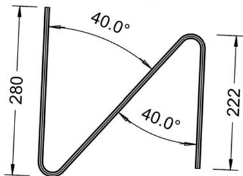
Figure 6 : détail suspente
