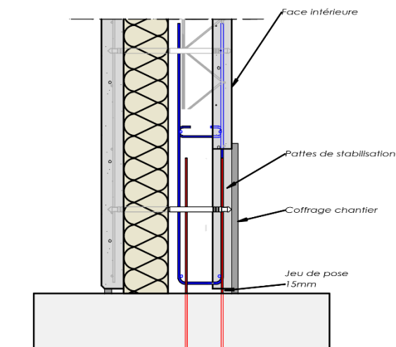
Figure 25 : Encastrement de l'(i)Premur A2C/radier → Liaison de type Er1
