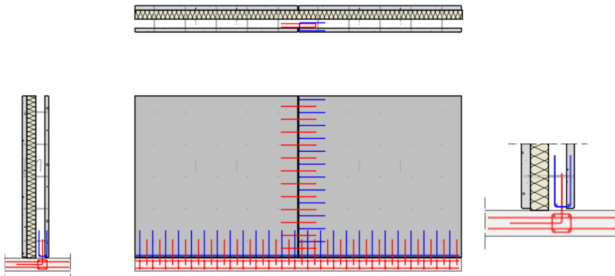
Figure 81 : poutre-voile reprenant la dalle – tirant dans l' (i) Prémur A2C
