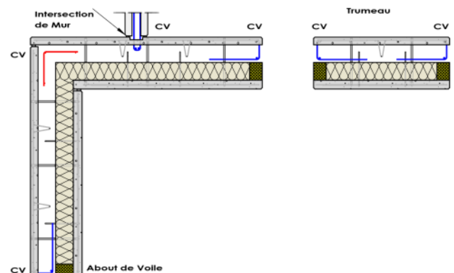
Figure 49 : Implantations des chaînages verticaux
