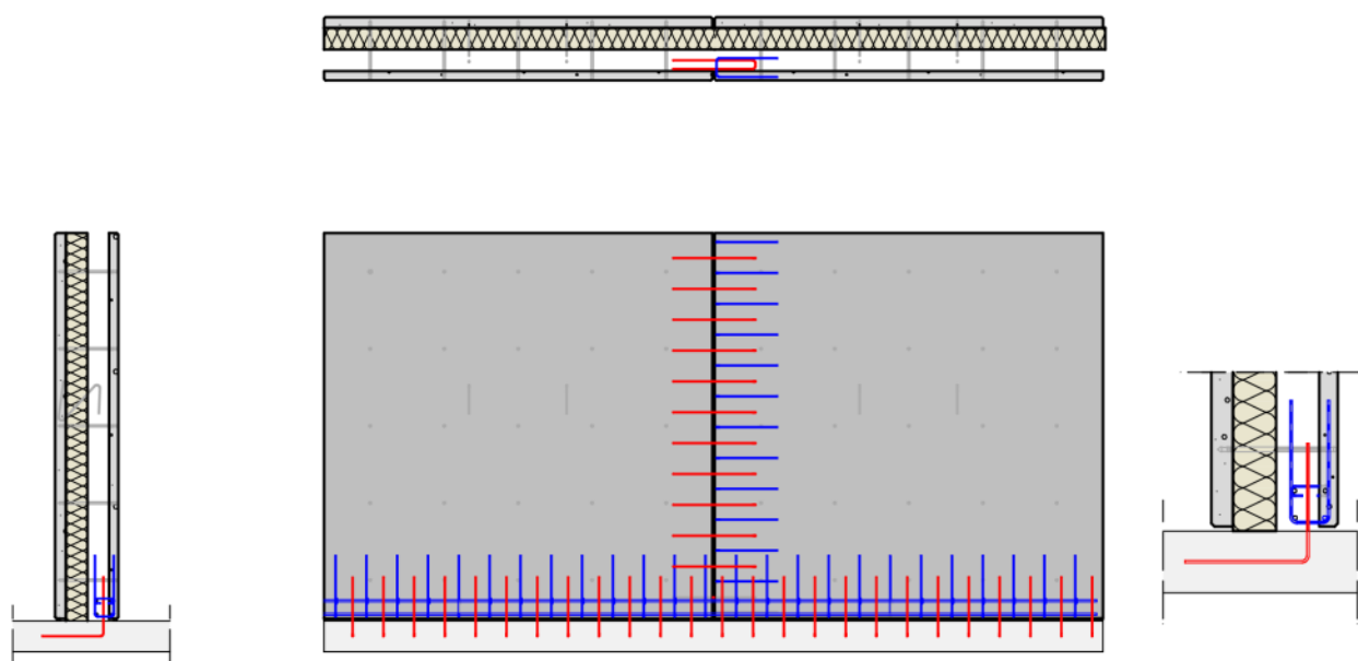
Figure 81 : poutre-voile reprenant la dalle – tirant dans l' (i) Prémur A2C
