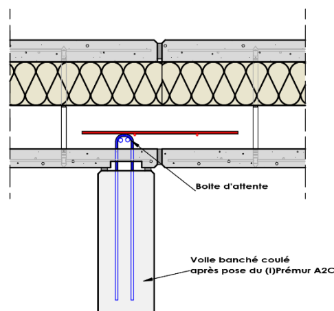
Figure 33 : Liaison en T entre un (i)Premur A2C et un mur coulé en place avec boîte d'attente.
