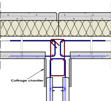
Figure 39 : Liaison verticale en T encastrée – Type Ev6
