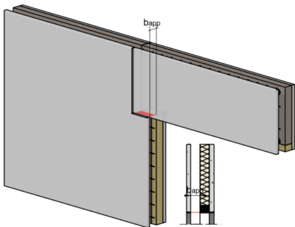
Figure 55 : Appui de poutre → Cas 2
