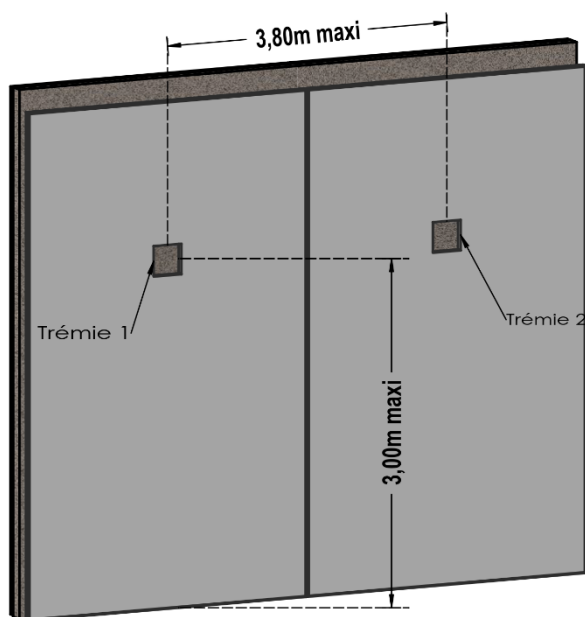
Figure 20 : Bétonnage par trémies
