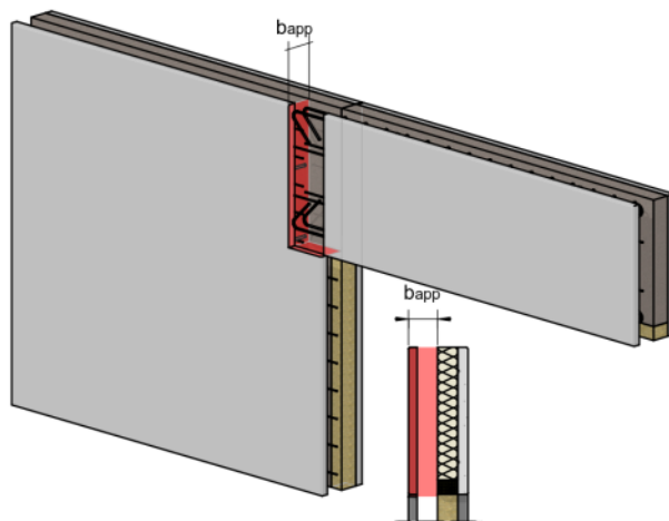
Figure 56 : Appui de poutre → Cas 3
