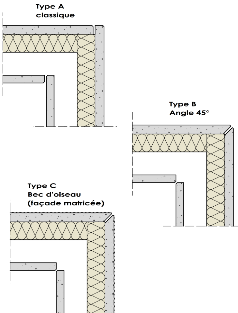
Figure 95 : Particularités des Liaisons en angle des (i)Premur A2C
