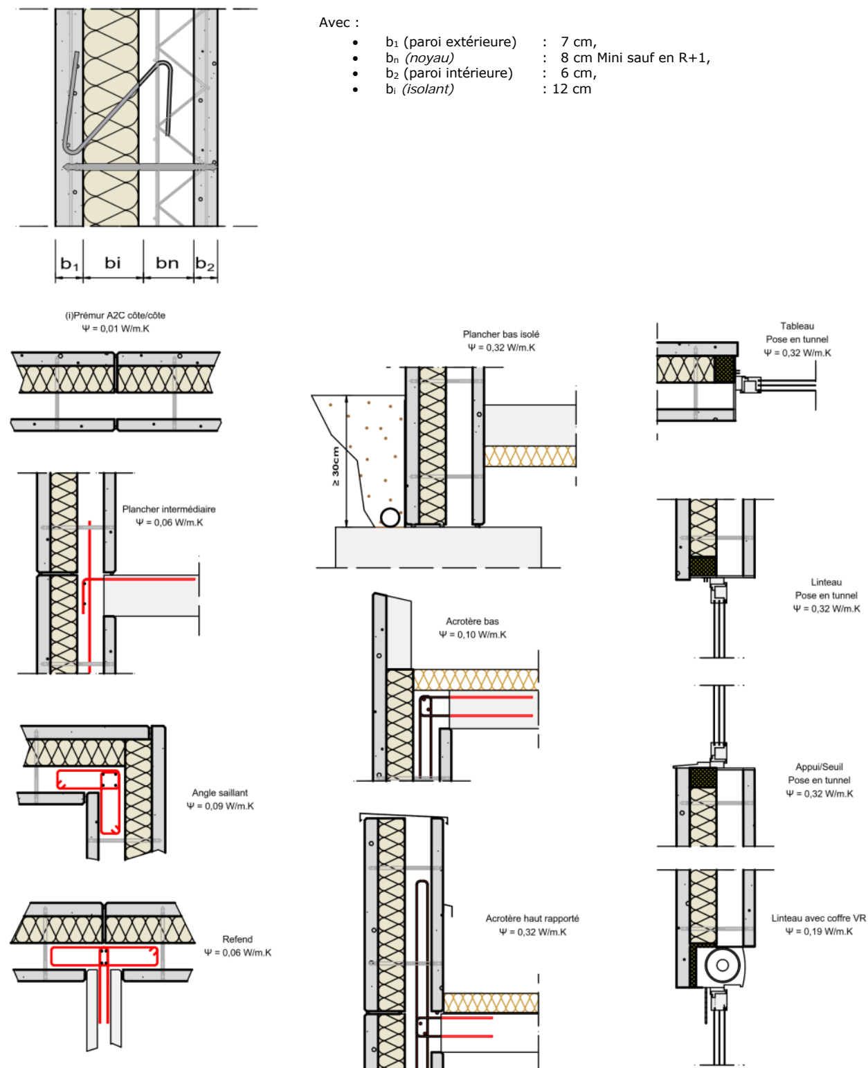
Figure 75 : coefficients de pertes linéiques
