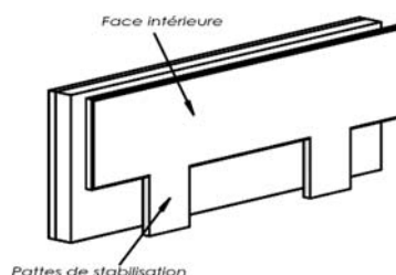
Figure 26 : Encastrement de l'(i)Premur A2C/radier → Liaison Er2
