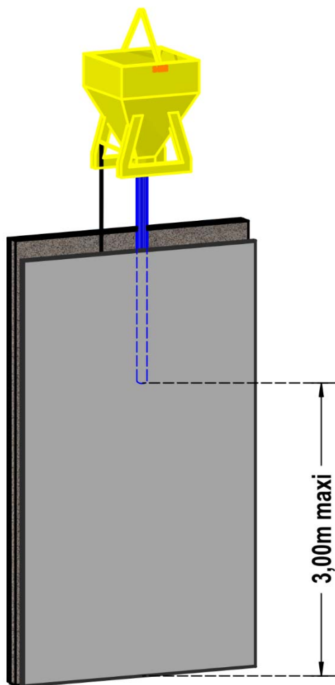
Figure 21 : Bétonnage par tube plongeant
