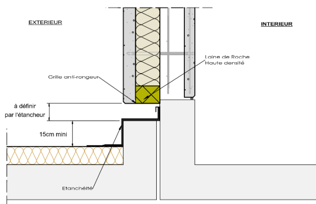
Figure 63 : Liaison (i)Premur A2C/Terrasse
