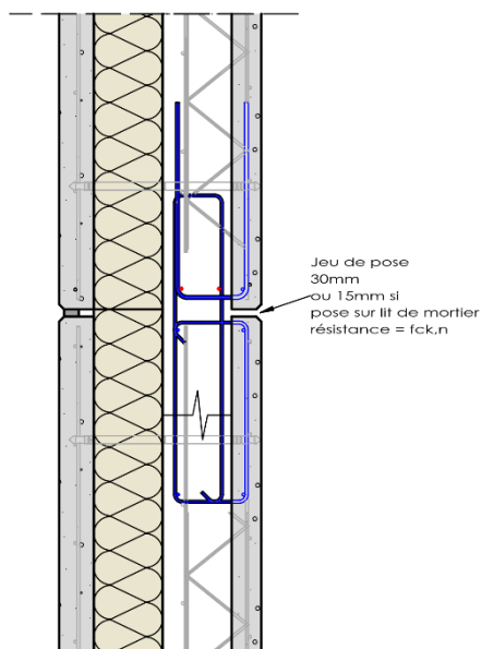
Figure 42 : Liaisons horizontales encastrées – Type Eh2
