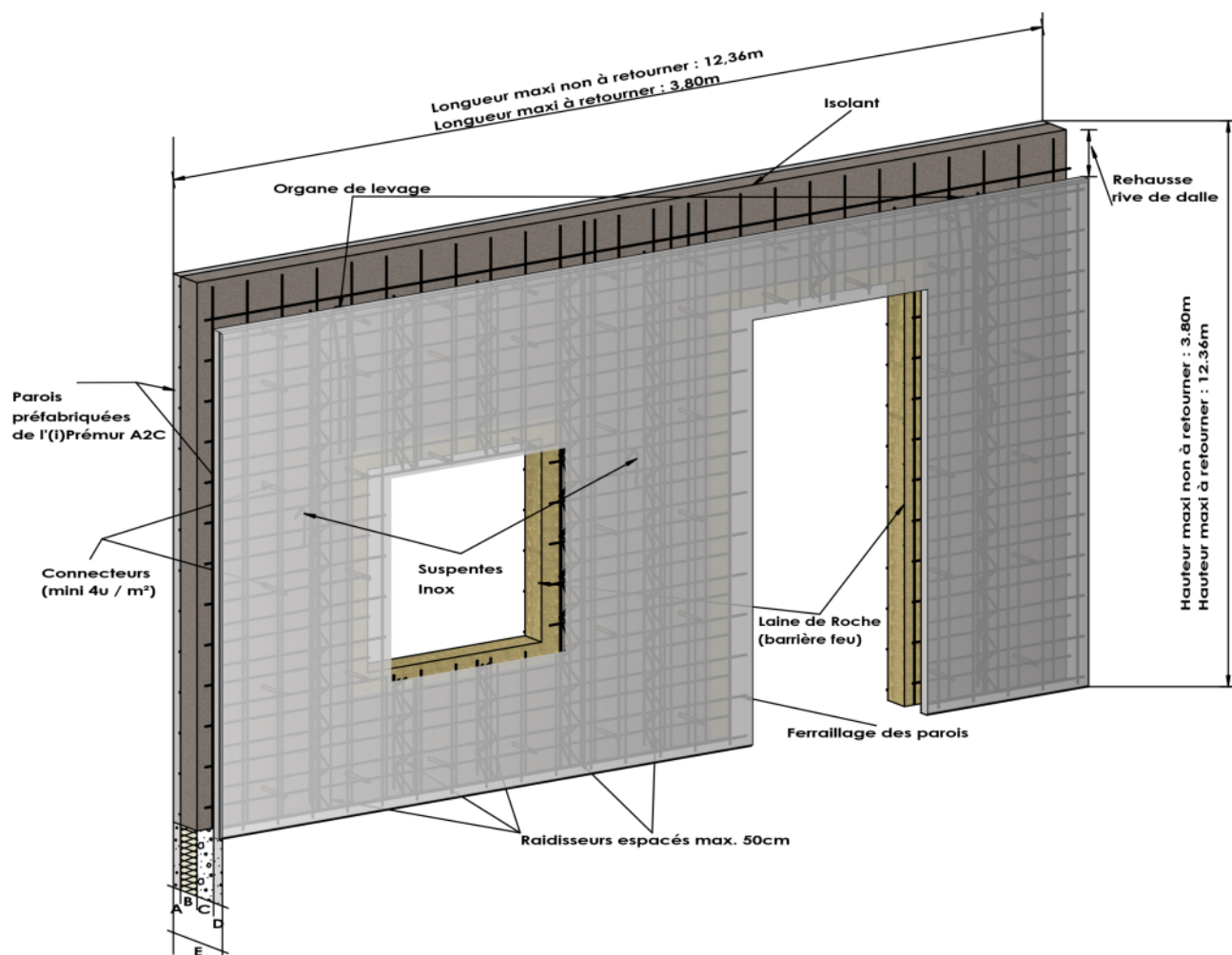
Figure 92 : Eclaté de l'(i)Premur A2
