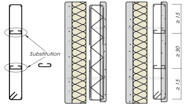
Figure 15 : Solution traditionnelle et de l'(i)Premur A2C
