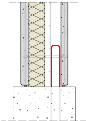
Figure 50 : Liaison en pied des murs courants
