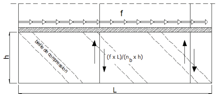
Figure 2 – Effort sollicitant dans le cas d'un contreventement avec reprise d'une charge linéaire horizontale (cas 2)
