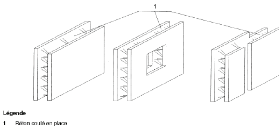
Figure 1 – Exemples de murs composites ou murs à coffrage intégré (source : NF EN 14992)
