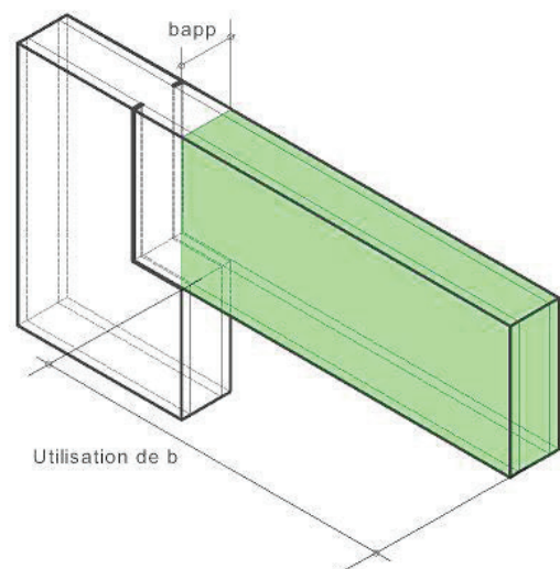
Figure A-26 – Appui de poutre – cas 3
